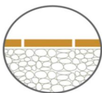
Сухая укладка на гальку
